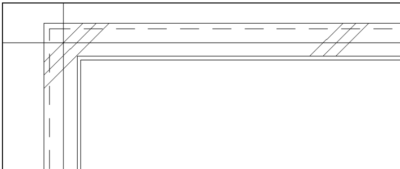
RCハッチ作図例
